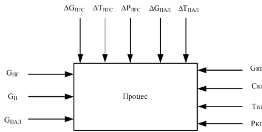
Рис. 2 – Схема об'єкта оптимізації
