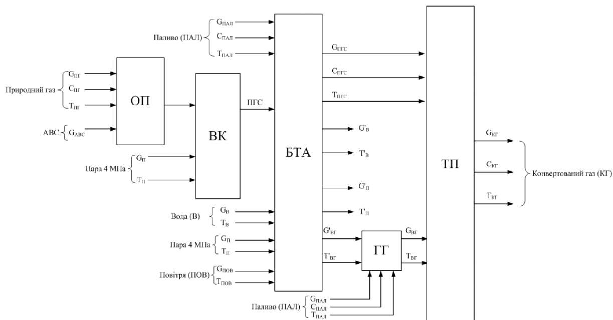
Рис. 1 – Структурно-параметрична схема процесу конверсії метану
