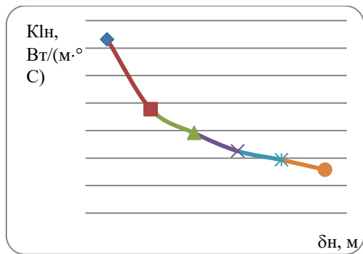
Рис. 3 – Залежність лінійного коефіцієнта теплопередачі K_{лн} від товщини шару накипу \delta_n на внутрішній поверхні труб горизонтального кожухотрубного теплообмінника
