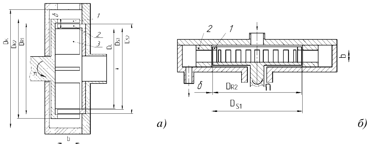
1 – ротор; 2 – статор; 3 – крилатка
