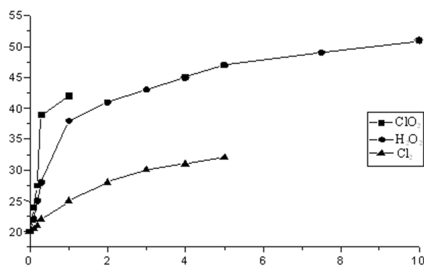
Рис. 6 – Залежність білості лляної целюлози, %, від витрати вибілювального реагенту, % а. с. ц.
