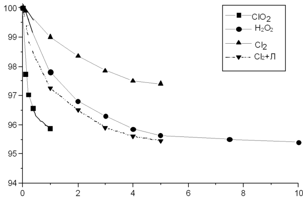
Рис. 1 – Залежність виходу целюлози, %, від витрати вибілювального реагенту, % а. с. ц.
