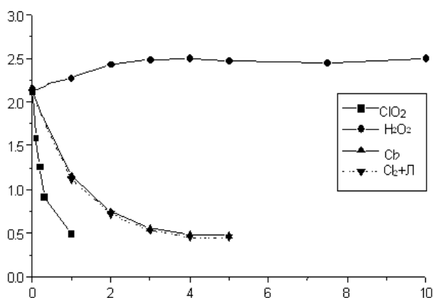
Рис. 5 – Залежність зольності целюлози, %, від витрати вибілювального реагенту, % а. с. ц.
