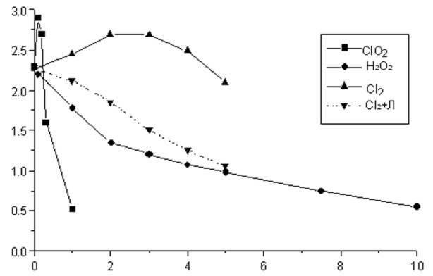
Рис. 2 – Залежність вмісту залишкового лігніну, %, від витрати вибілювального реагенту, % а. с. ц.
